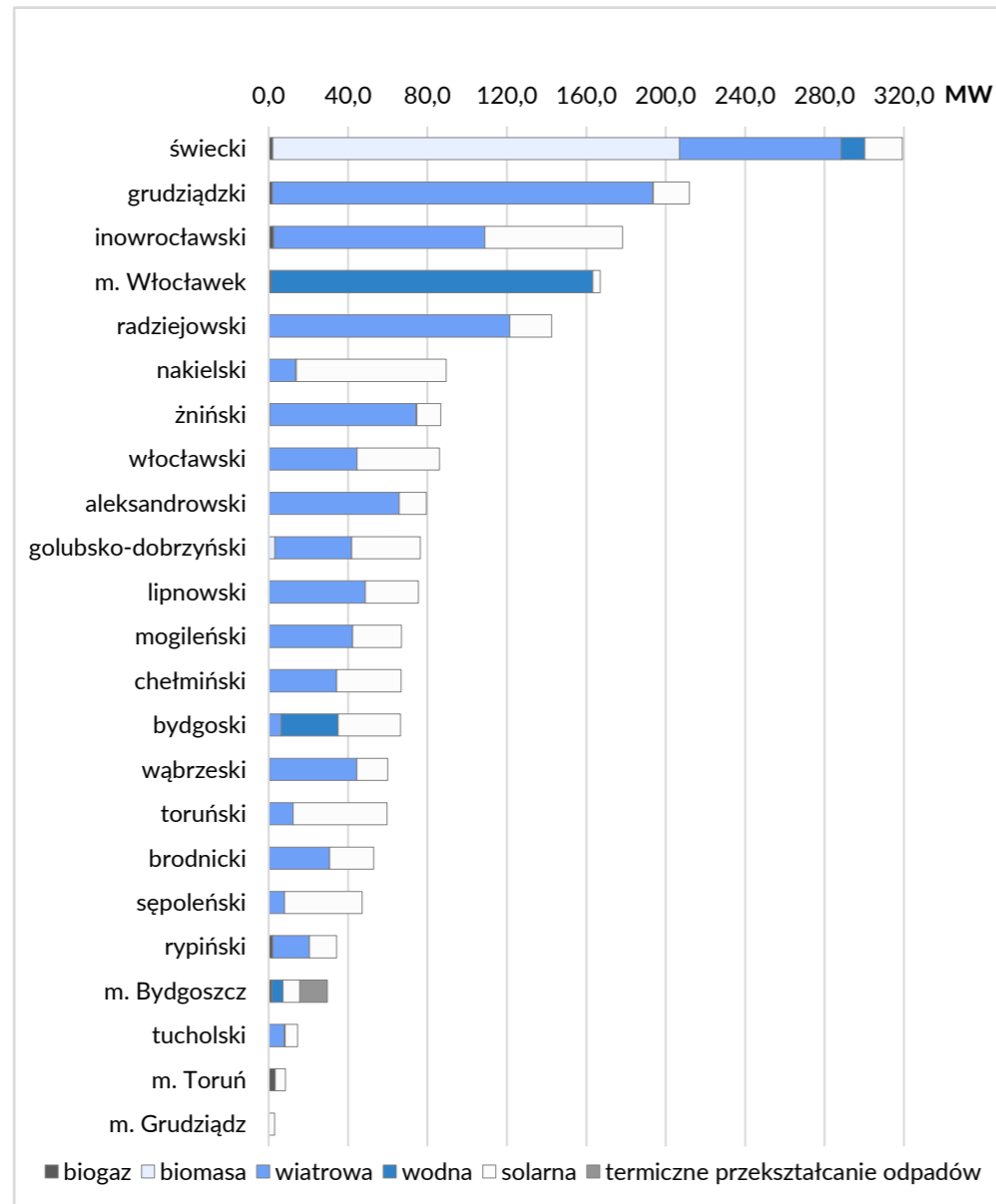
Moc zainstalowana poszczególnych instalacji wytwórczych OZE na terenie powiatów województwa kujawsko-pomorskiego bez mikroinstalacji według stanu na 30 września 2025 r. (MW).
